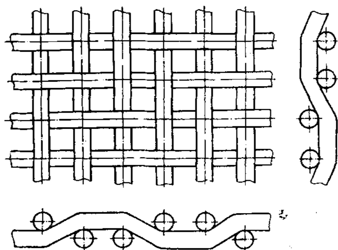
图2 斜纹编织
