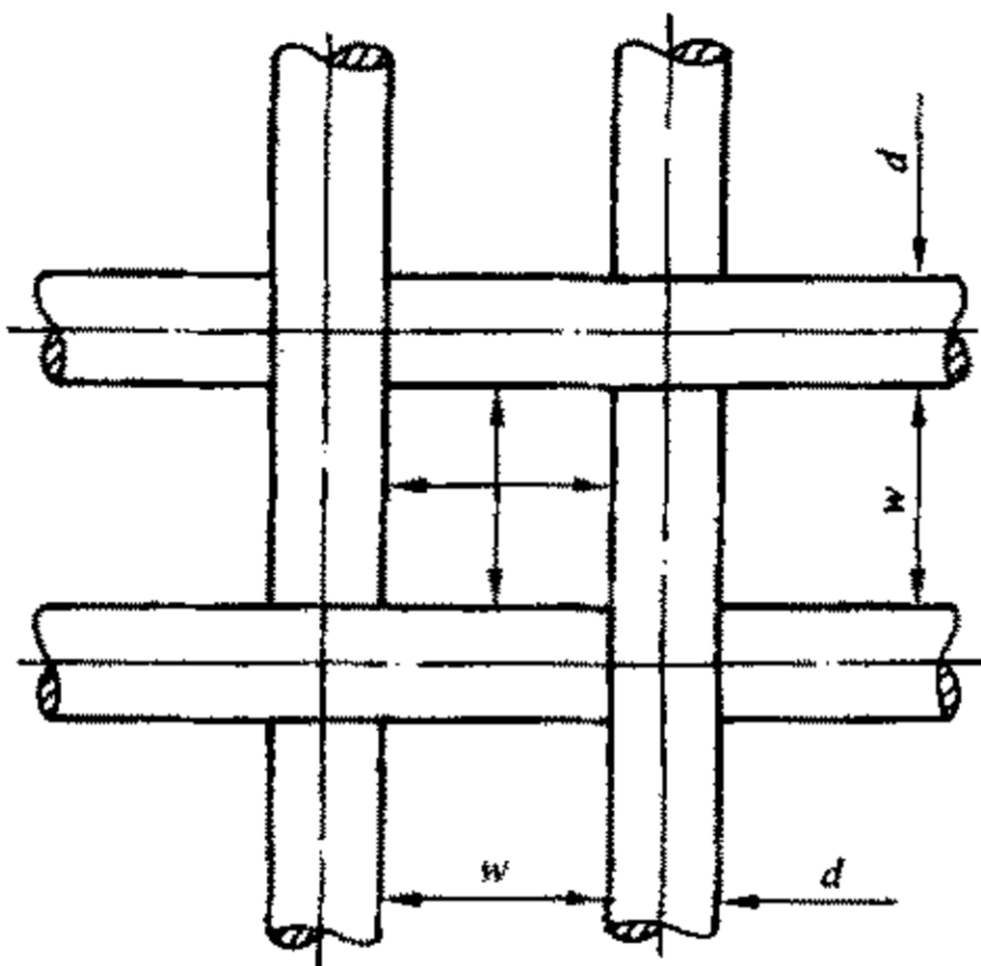
图 3 网孔尺寸和丝径
